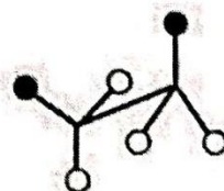
gauche conformation
